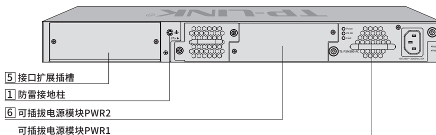
图1-14 TL-SH7452后面板示意图
