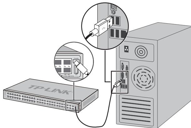
图3-5 Type-C Console端口连接示意图
