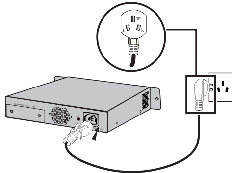
图3-10 TL-RPS150连接电源线示意图
