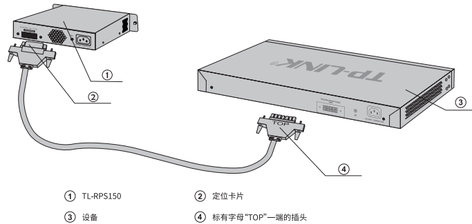
图3-9 连接设备和TL-RPS150示意图
