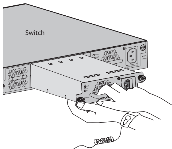
图3-8 安装电源模块示意图（以TL-SH7452为例）
