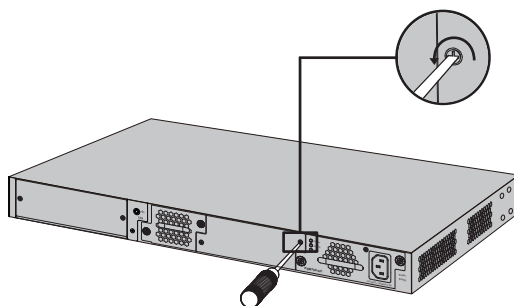
图3-7 移除保护面板示意图
