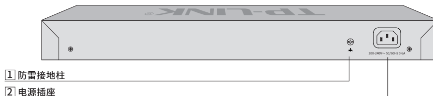
图1-8 TL-SH6428后面板示意图
