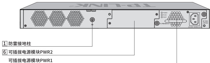
图1-13 TL-SH6654GF后面板示意图
