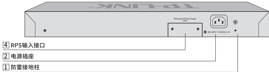
图1-12 TL-SH7428F后面板示意图
