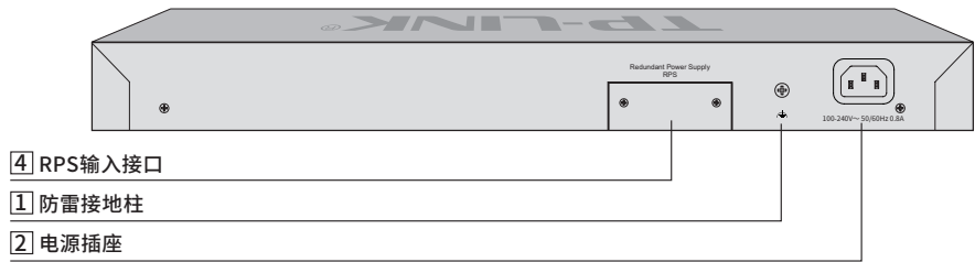
图1-11 TL-SH7428后面板示意图
